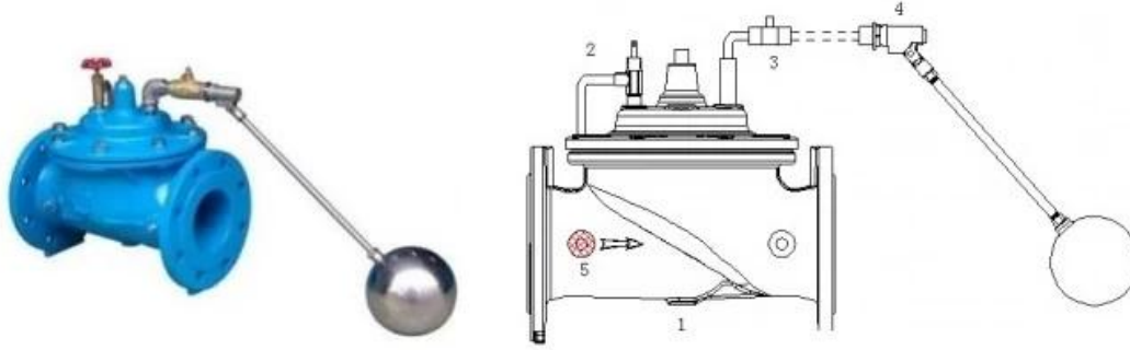
1. كروية العائم. 2. ذراع العائم. 3. غشاء. 4. مقعد الصمام. 5. ذراع العائم.
