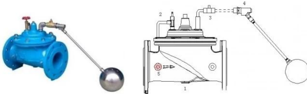
1. Hauptventil 2. Nadelventil 3. Ballventil 4. Schwimmerpilot 5. Sieb
