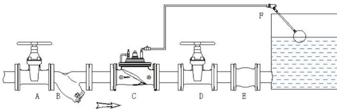
A. Shut Off Ventil B.y Sieb C. Float -Kontrollventil D. Shut Off Ventil E. SOFT FOINK F.Float Pilot
