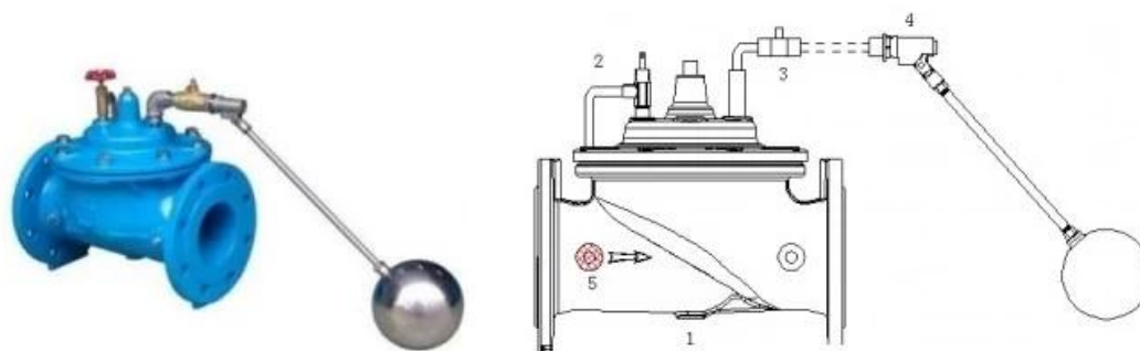
1. Válvula principal 2. Válvula de aguja 3. Válvula de bola 4. Piloto de flotador 5. Filtro
