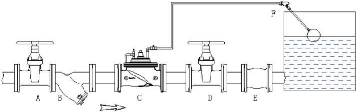
A.手輪 B.Y型過濾器 C.閥門 D.手輪 E.管道 F.浮球閥
