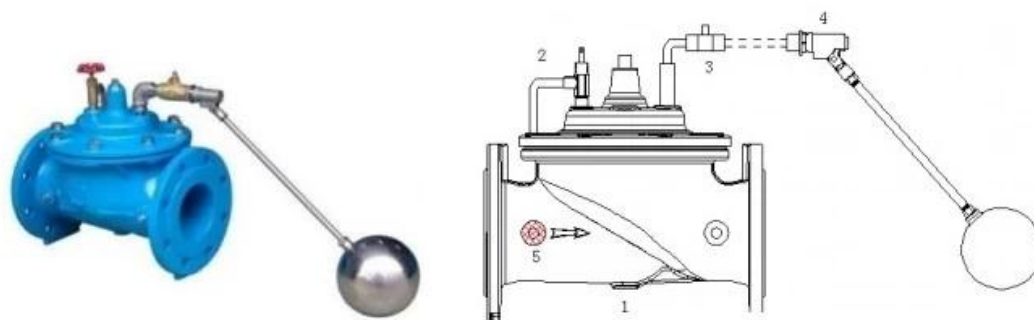
1. Основной клапан 2. Игольчатый клапан 3. Шаровой клапан 4. Плотный пилот 5. Ситец
