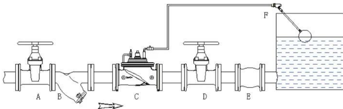
A. 截止閘門 B. Y C. 浮球閘門 D. 截止閘門 E. 閘門 F. 浮球閘門
